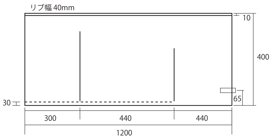
FLG1800×600 用ろ過槽 1200×400×400H t=5
