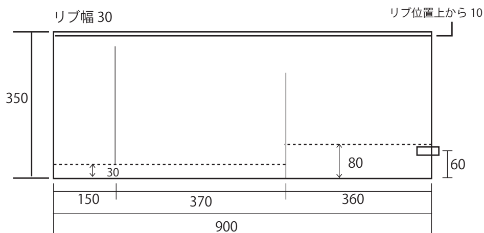
FLG 1200×450 用 900×280×350 t=4
