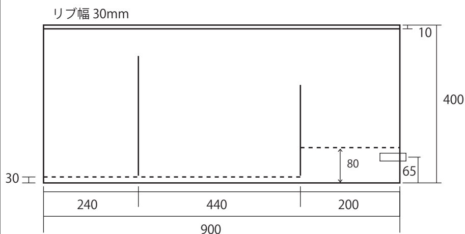
FLG1200×600 用ろ過槽 900×400×400H t=4
